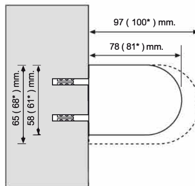
INSTALACIÓN A PARED FACE FIX
