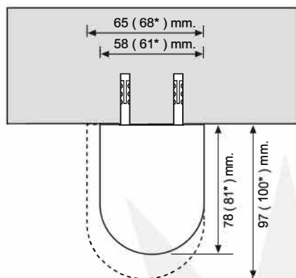
INSTALACIÓN A TECHO TOP FIX
