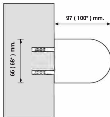
INSTALACIÓN A PARED FACE FIX
