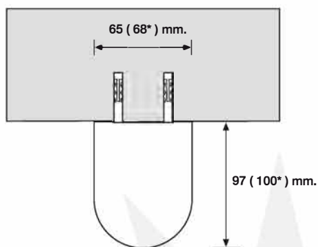
INSTALACIÓN A TECHO TOP FIX
