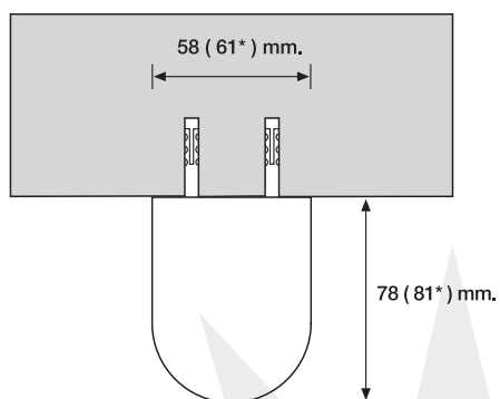
INSTALACIÓN A TECHO TOP FIX
